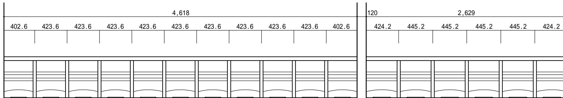
西側手摺(内観図) 1/30
